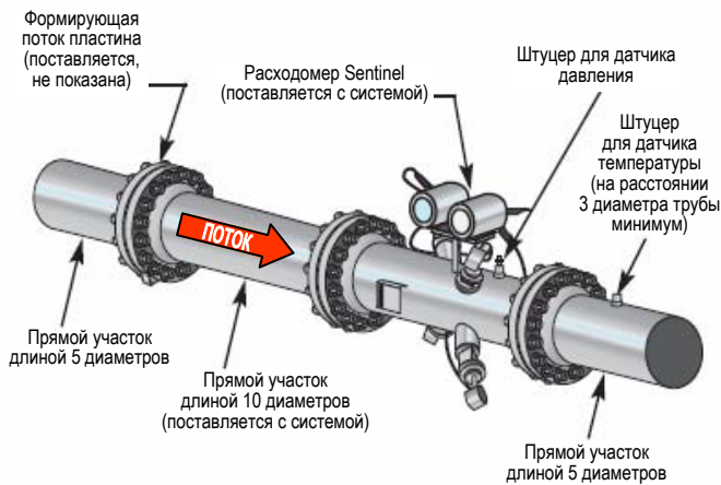
Установка Sentinel для однонаправленного потока
