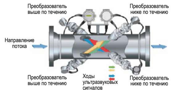
Времяимпульсная технология измерения расхода
